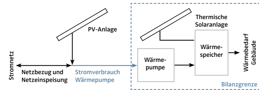
Messbilanz Wärmepumpe
